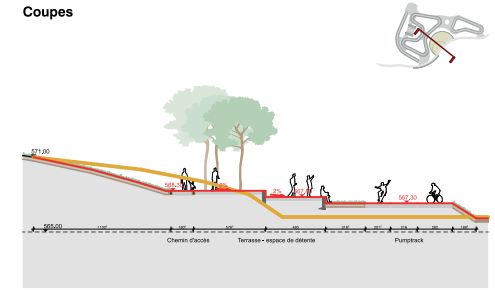
Coupes
